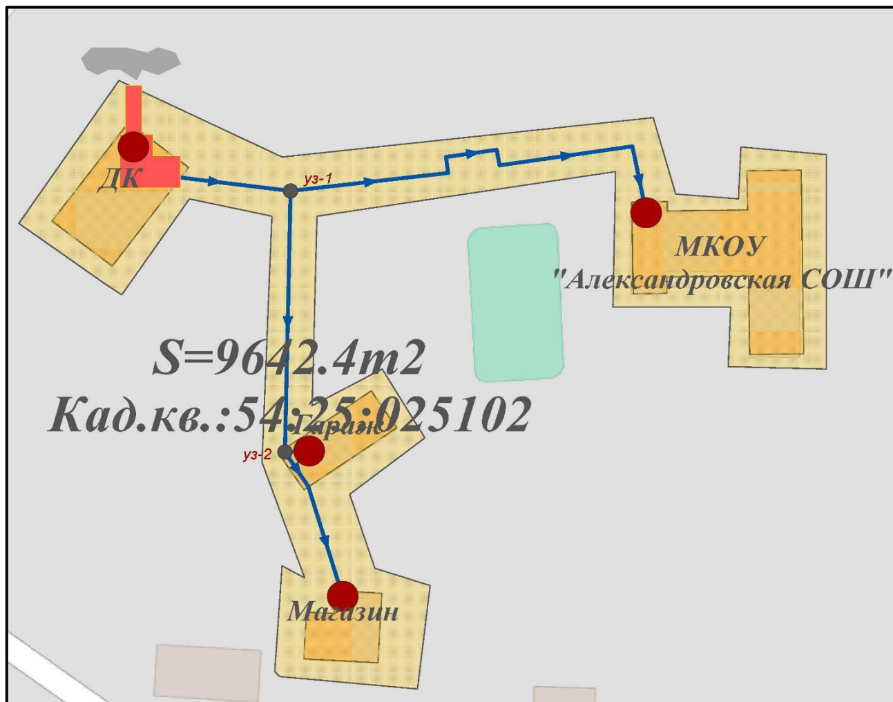
Рисунок 1.1.3.1 – Зона действия отопительной котельной
