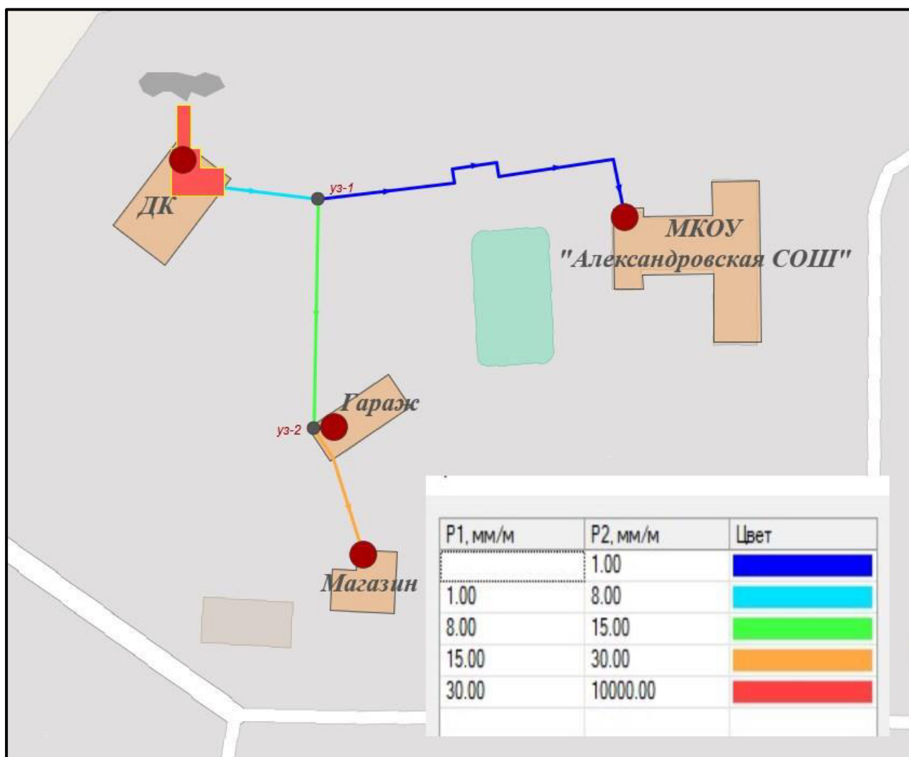
Рисунок 4.2.1 – Пропускная способность теплосетей (в цвете)
