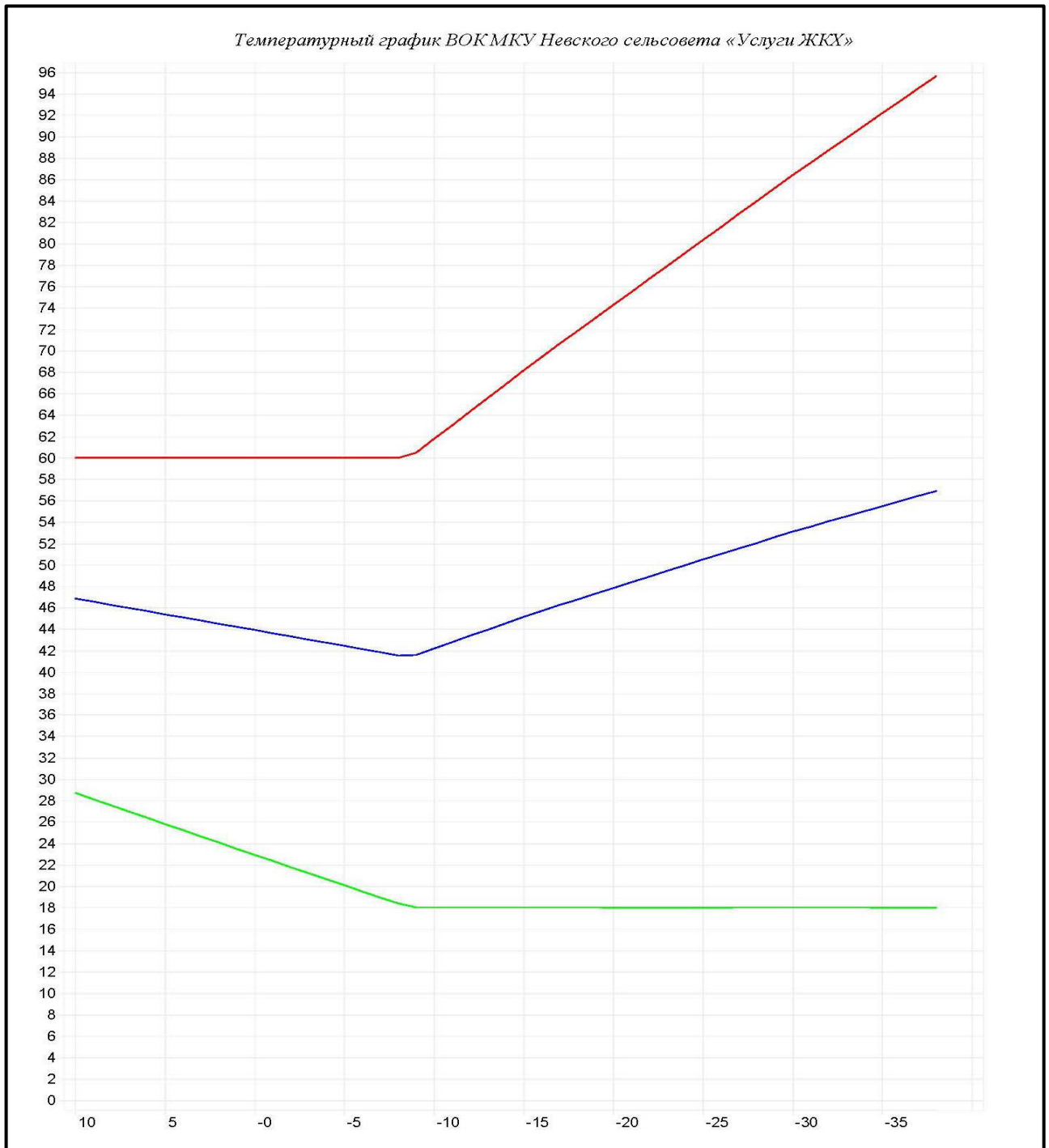
Рисунок 5.8.1 – Расчет отпуска тепловой энергии для котельной Невского сельсовета Убинского района в течение года при температурном графике 95-70 °С
