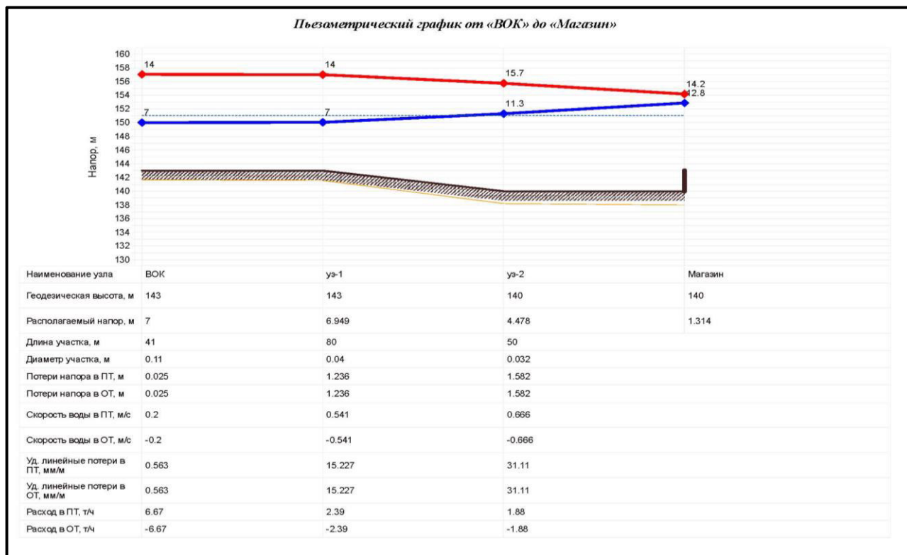
Рисунок 1.3.8.1 – Пьезометрический график по пути: ВОК –Магазин
