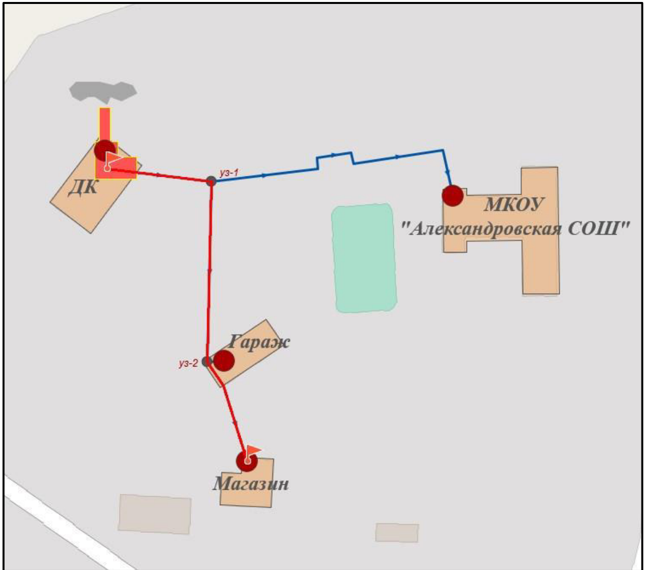
Рисунок 1.3.8.2 – Путь для пьезографика: ВОК –СОШ
