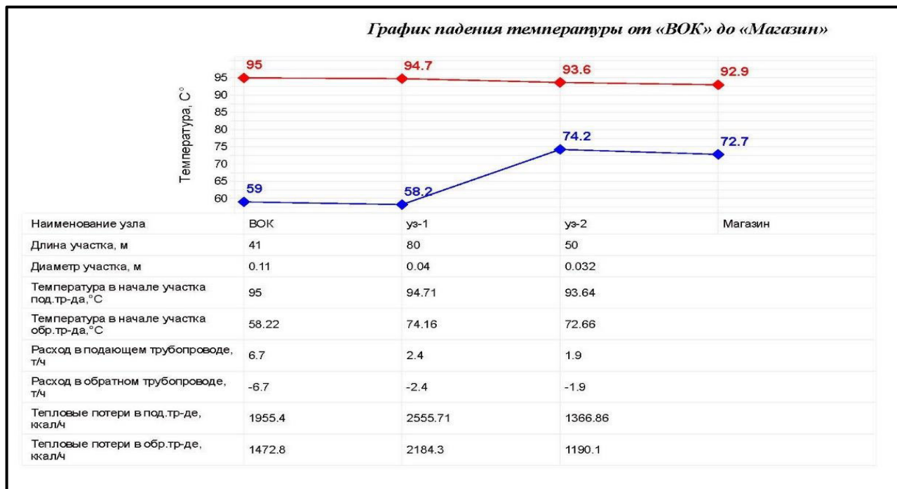
Рисунок 1.3.8.3 – График падения температуры от ВОК –Магазин
