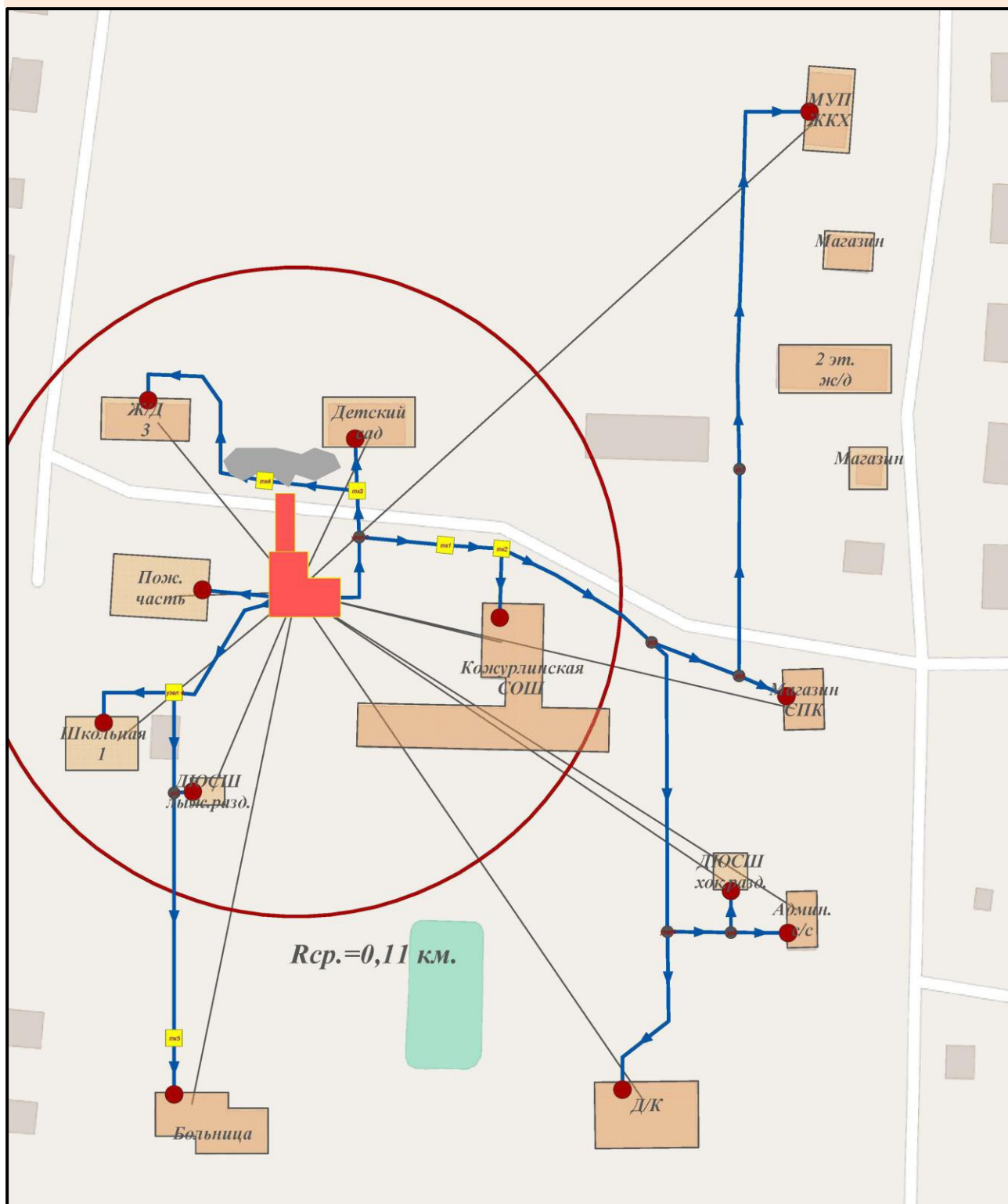
Рисунок 2.5.1 – РЭС Котельной БМК
