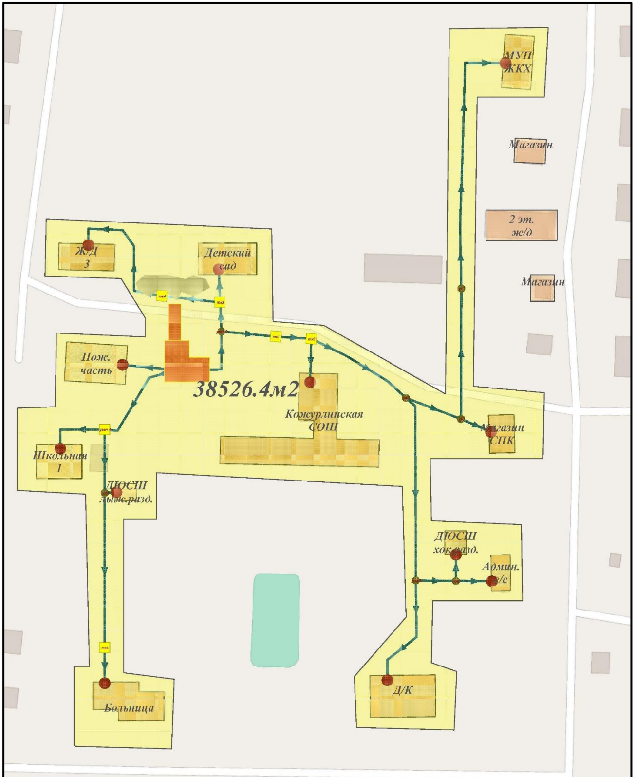
Рисунок 1.1.3.1 – Зона действия Котельной БМК
