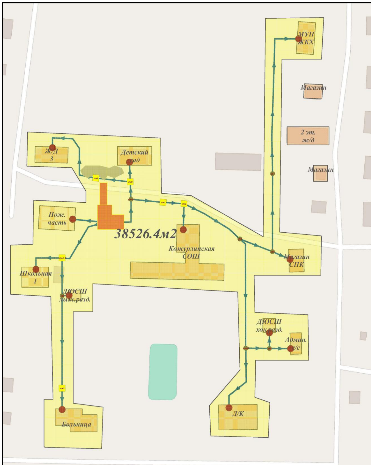
Рисунок 2.4.1 – Зона действия Котельной БМК
