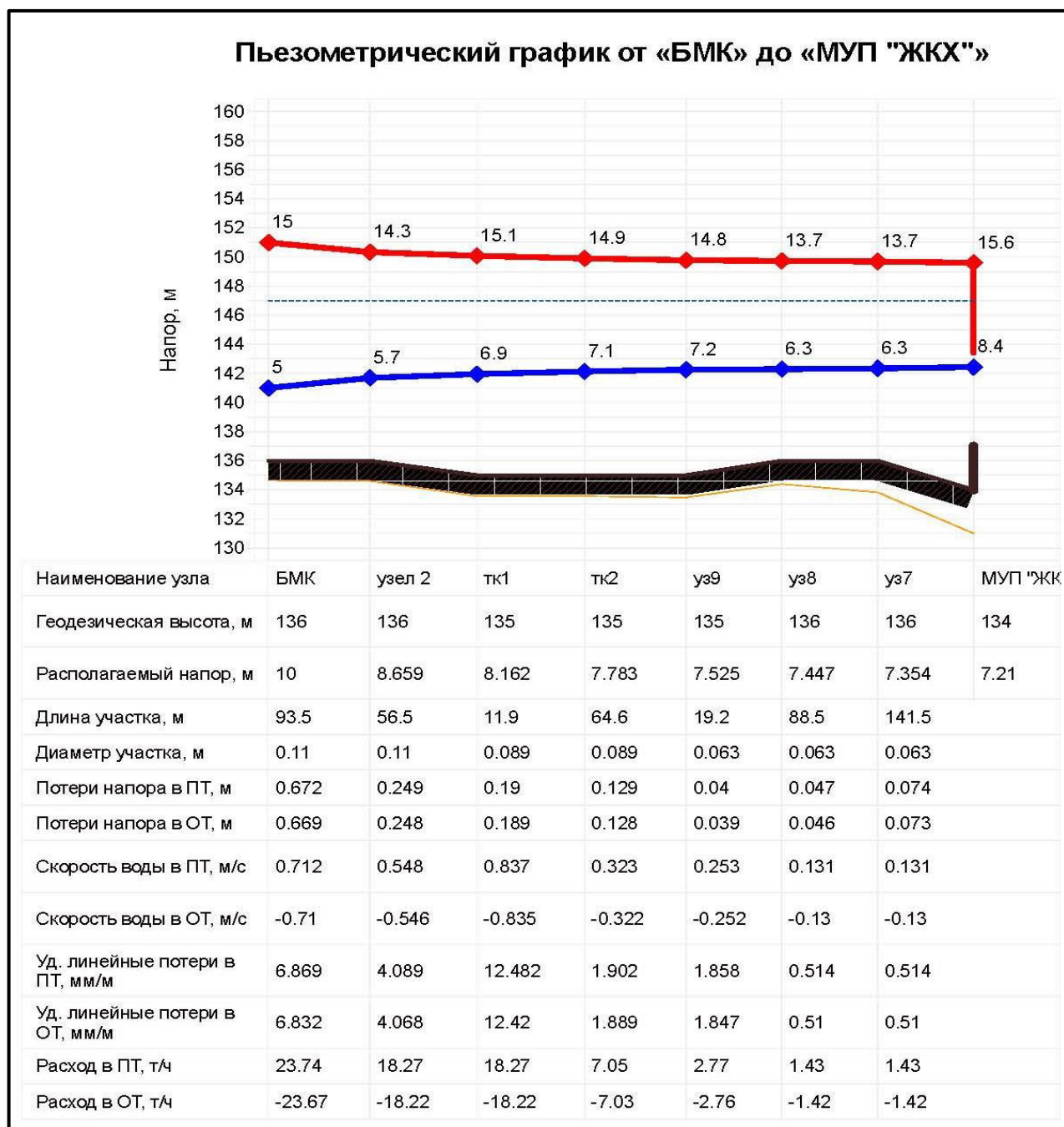
Рисунок 1.3.8.2 – Пьезометрический график по пути: БМК – МУП «ЖКХ»
