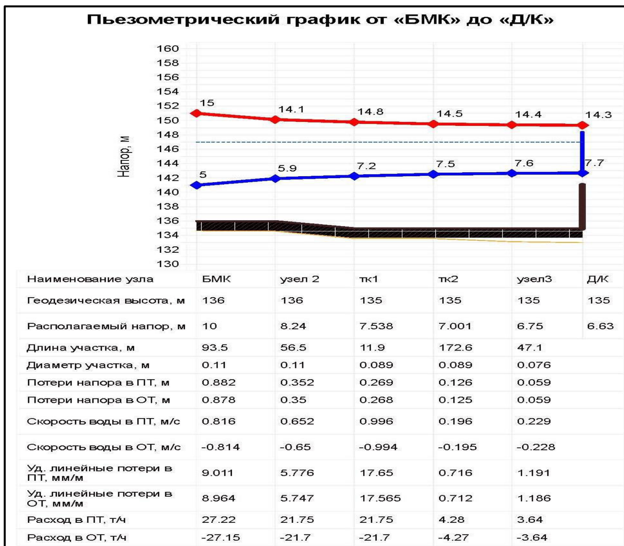
Рисунок 1.3.8.1 – Пьезометрический график по пути: БМК – Д/К
