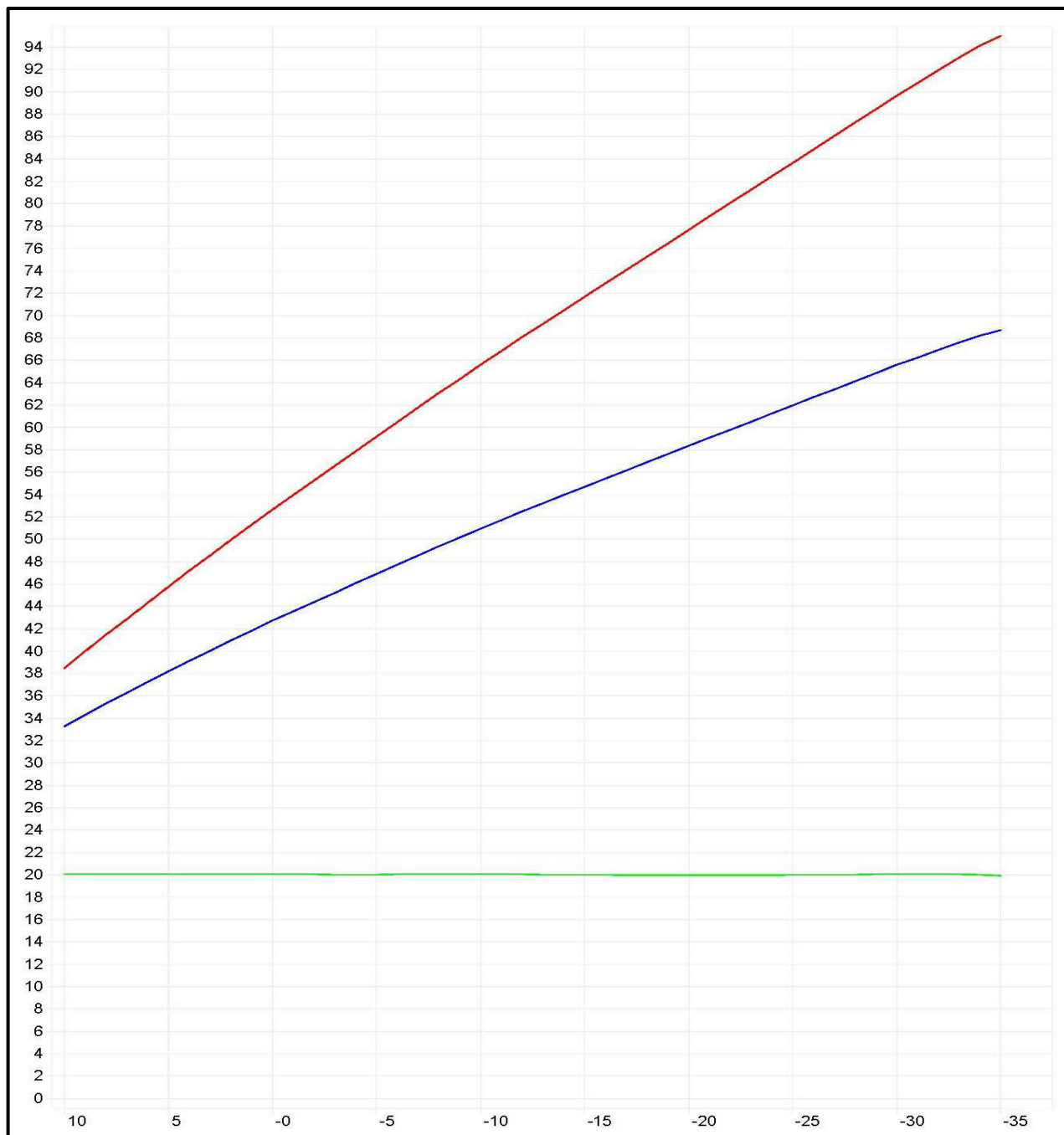
Рисунок 1.2.7.1 – График изменения температур теплоносителя 95–70 °С
