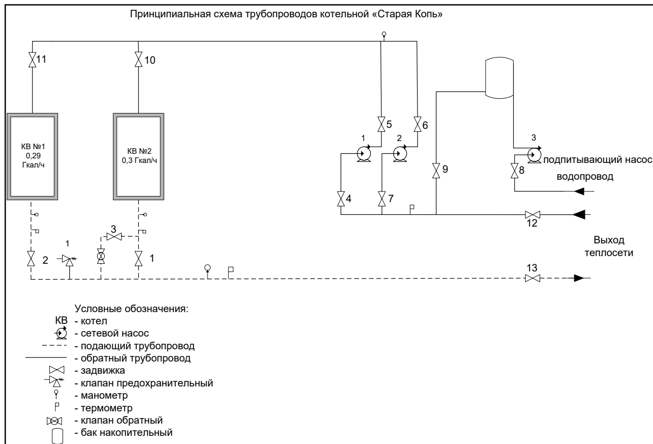
Рисунок 1.2.6.1 – Принципиальная тепловая схема котельной с водогрейными котлами
