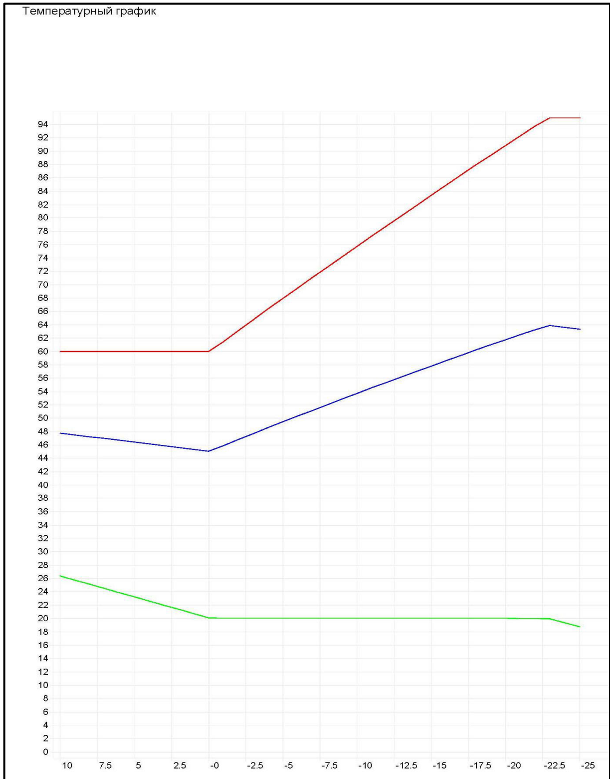
Рисунок 5.8.1 – Расчет отпуска тепловой энергии для котельной Колмаковского сельсовета Убинского района в течение года при температурном графике 95-70 °С
