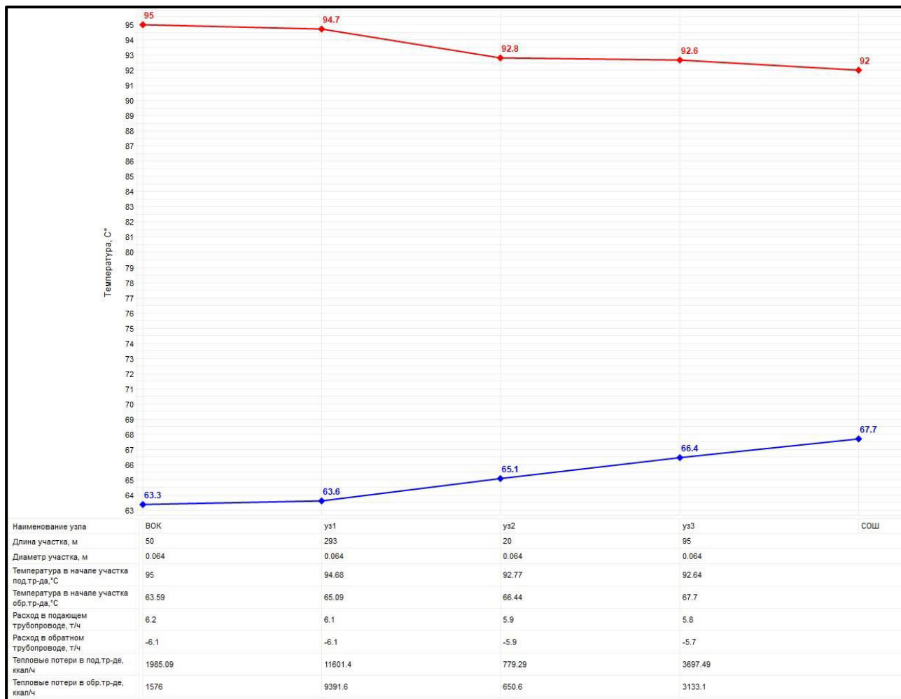
Рисунок 1.3.8.3 – График падения температуры от ВОК –СОШ
