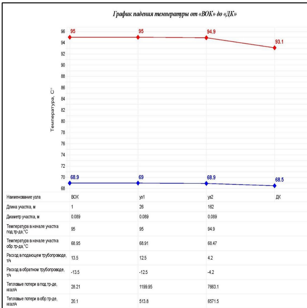
Рисунок 1.3.8.3 – График падения температуры от ВОК –ДК
