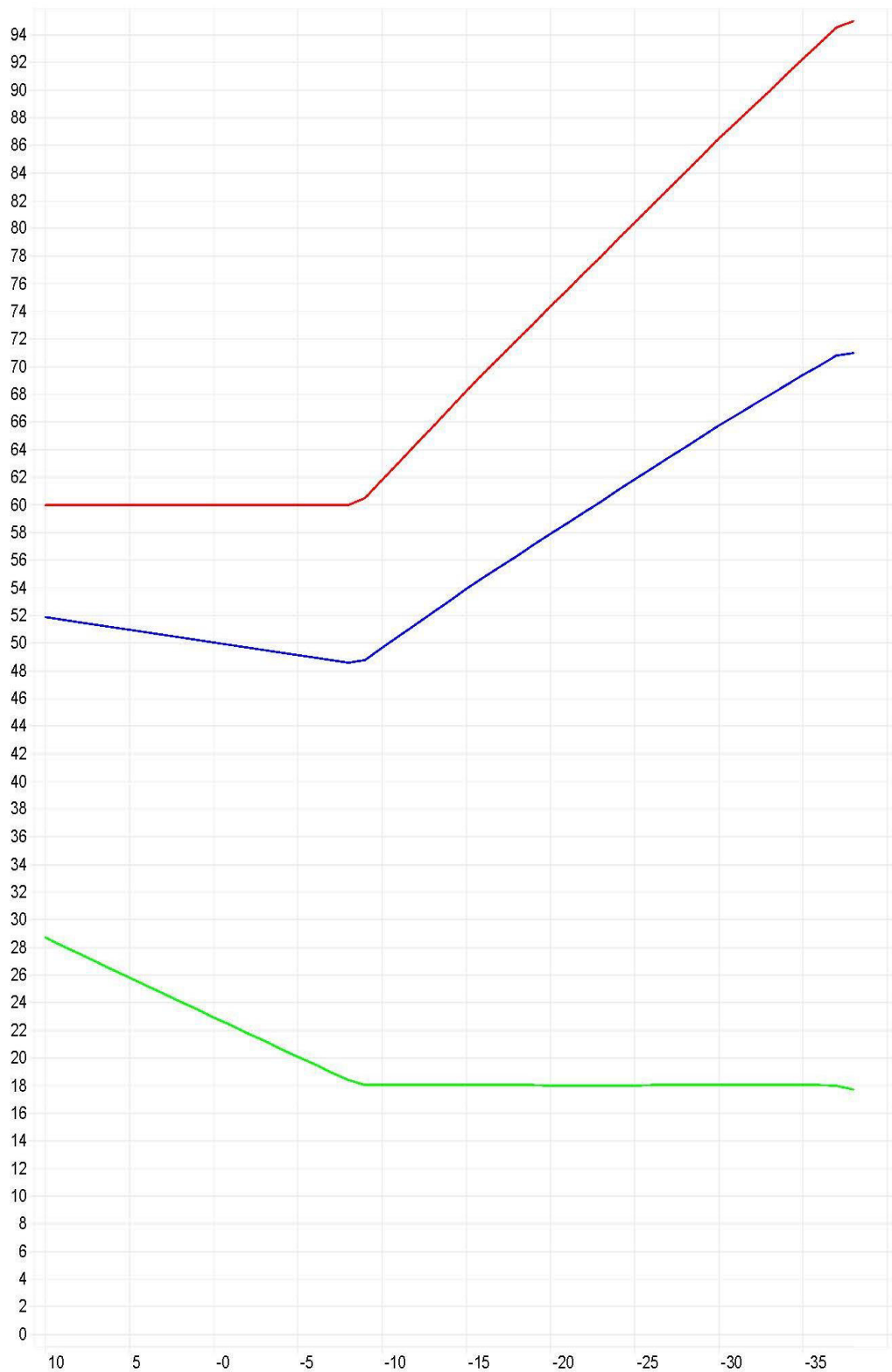
Рисунок 1.2.7.1 – График изменения температур теплоносителя 95–70 °С
