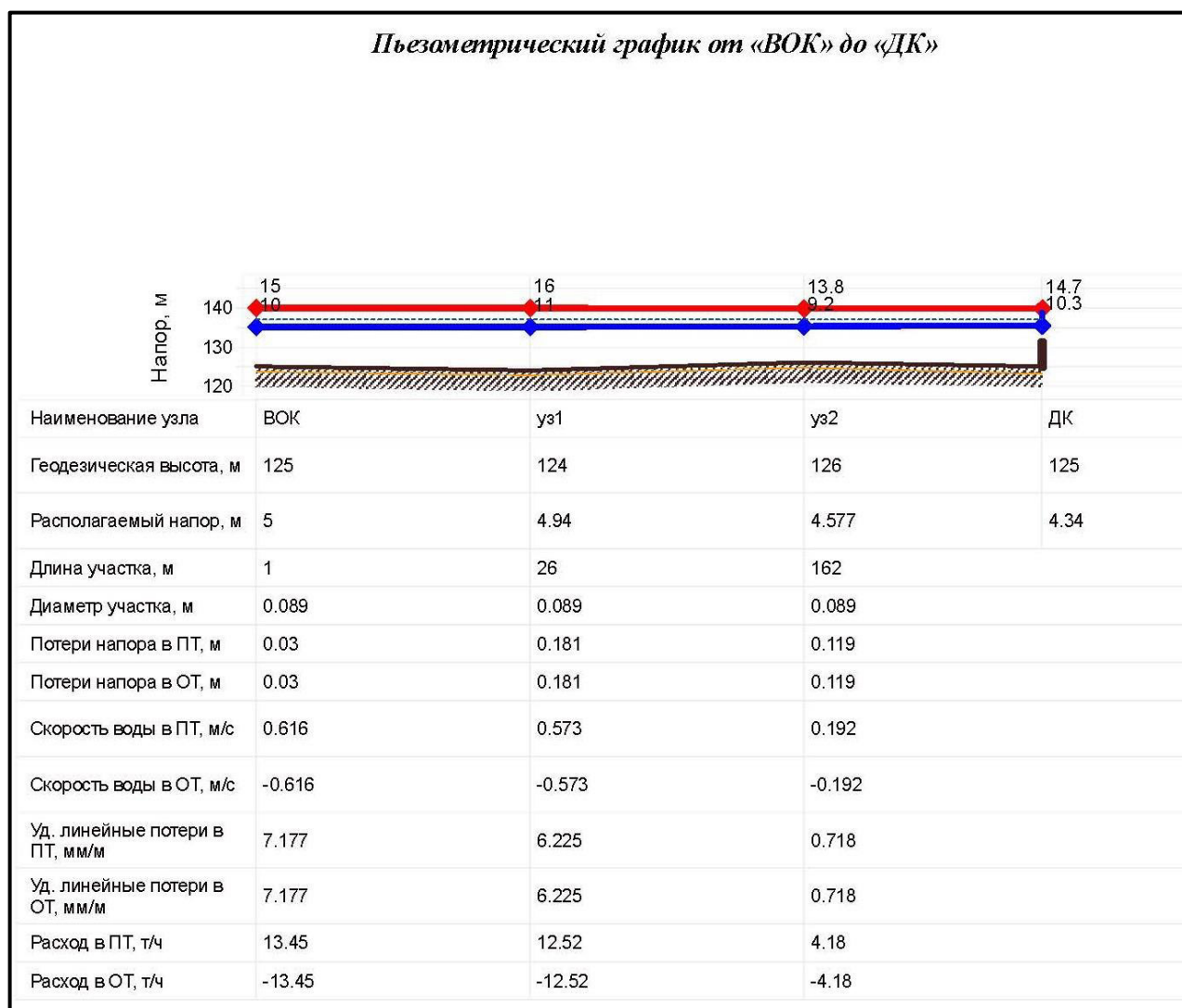
Рисунок 1.3.8.1 – Пьезометрический график по пути: ВОК – ДК
