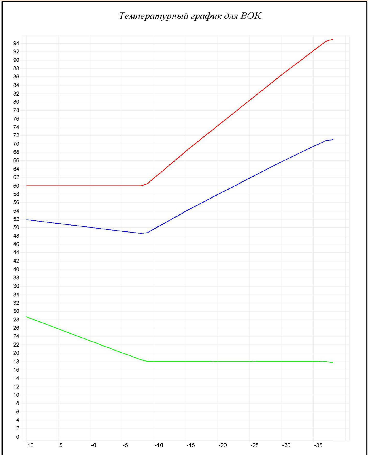
Рисунок 5.8.1 – Расчет отпуска тепловой энергии для котельной Гандичевского сельсовета Убинского района в течение года при температурном графике 95-70 °С
