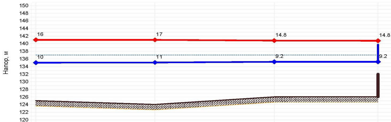
Пьезометрический график от «ВОК» до «Школа»
