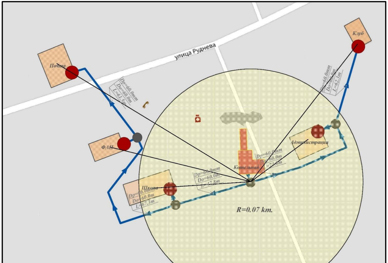
Рисунок 2.5.1 – РЭС Муниципальной котельной
